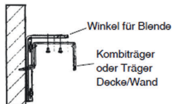
Abb.3 Kombiträger an Winkel für Blende
